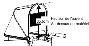
Hauteur de l'auvent Au-dessus du matériel Le matériel se monte sur la partie verticale de la canne arrière
